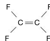
(d) tetrafluoroethene
