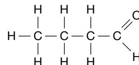
butanal
