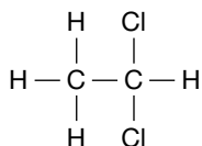
1,1-dichloroethane, \text{CH}_3\text{CHCl}_2
