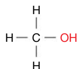
\text{CH}_3\text{OH} methanol
