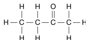
butanone
