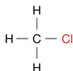
\text{CH}_3\text{Cl} chloromethane
