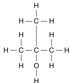
2-methylpropan-2-ol
