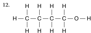
butan-1-ol
