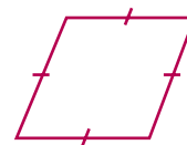
Rhombus
